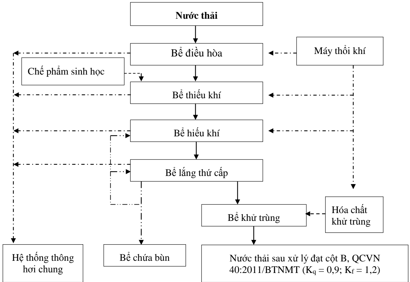
Sơ đồ công nghệ xử lý của hệ thống xử lý nước thải tập trung
