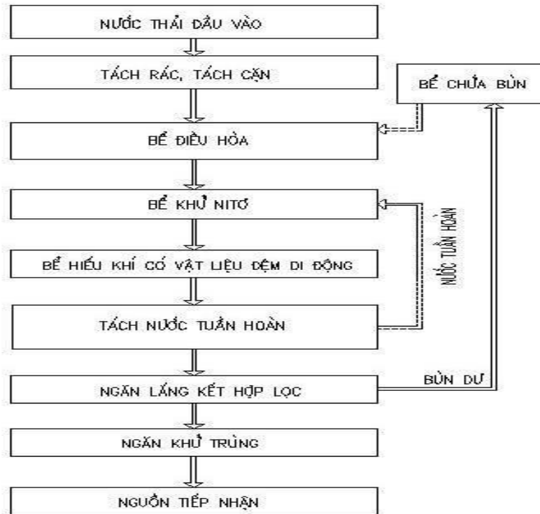
Sơ đồ công nghệ xử lý nước thải
